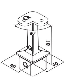
Käsijohteen kannake 90°
