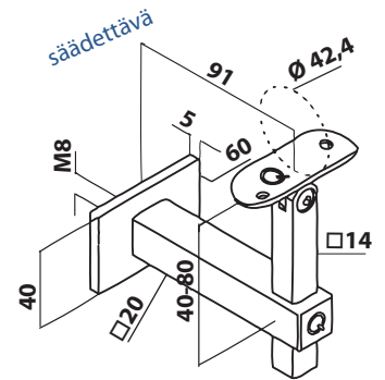
Käsijohteen kannake seinään
