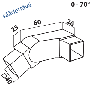
Käsijohteen kulma
