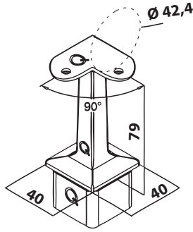
Käsijohteen kannake 90°
