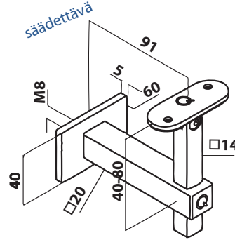
Käsijohteen kannake seinään
