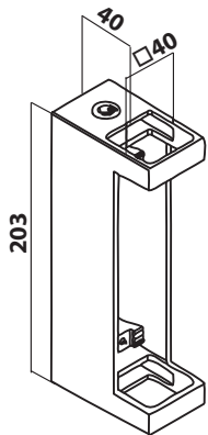
Kaidetolpan sivukiinnike
