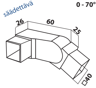
Käsijohteen kulma
