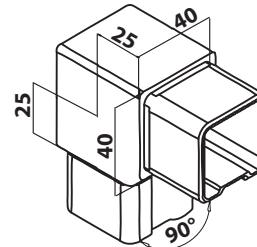
Käsijohteen kulma
