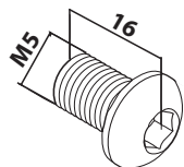
Ruuvi käsijohteen kannakkeille sisälle 93.0511.516.13 ulos 93.0511.516.14
