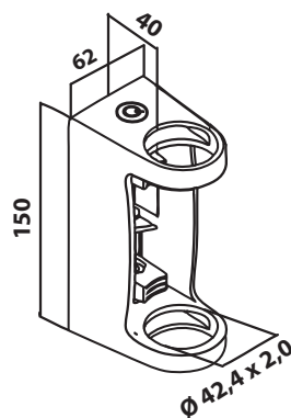
Kaidetolpan sivukiinnike sisälle 13.0557.042.12 ulos 14.0557.042.12
