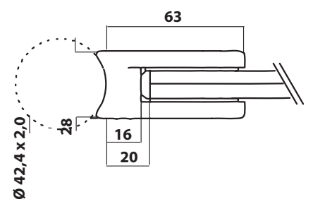
Kaidehela 8mm lasille sisälle 10.2208.042.19 (RST-efekti) sisälle 13.2208.042.12 ulos 14.2208.042.12
