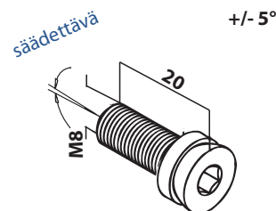
Ruuvi kaideheloille sisälle 93.0900.820.15 (sinkitty) sisälle 93.0900.820.13 ulos 93.0900.820.14
