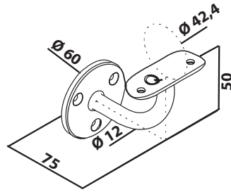
Käsijohteen kannake seinään sisälle 13.0112.042.12 ulos 14.0112.042.12
