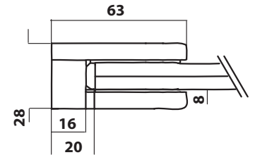
Käsijohteen liitos sisälle 13.0790.242.12 ulos 14.0790.242.12
