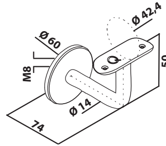
Käsijohteen kannake seinään sisälle 13.0111.042.12 ulos 14.0111.042.12
