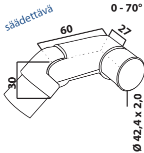
Käsijohteen kulma sisälle 13.0317.242.12
