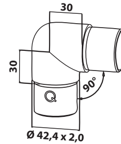
Käsijohteen kulma sisälle 13.0303.242.12 ulos 14.0303.242.12
