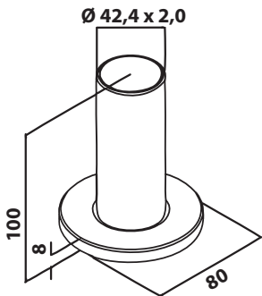
Kaidetolpan jalka sisälle 13.0946.242.12
