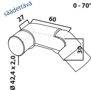
Käsijohteen kulma sisälle 13.0318.242.12
