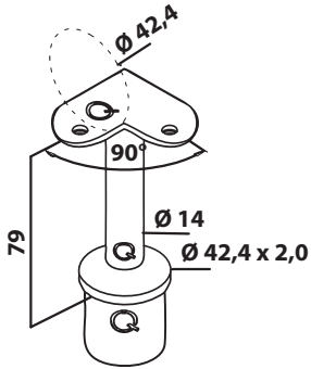
Käsijohteen kannake 90° sisälle 13.0710.842.12 ulos 14.0710.842.12
