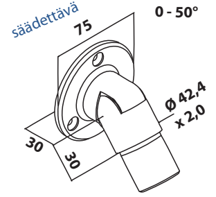
Käsijohteen pääty seinään sisälle 13.0506.242.12
